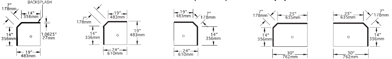
model #ICWB-19/19
